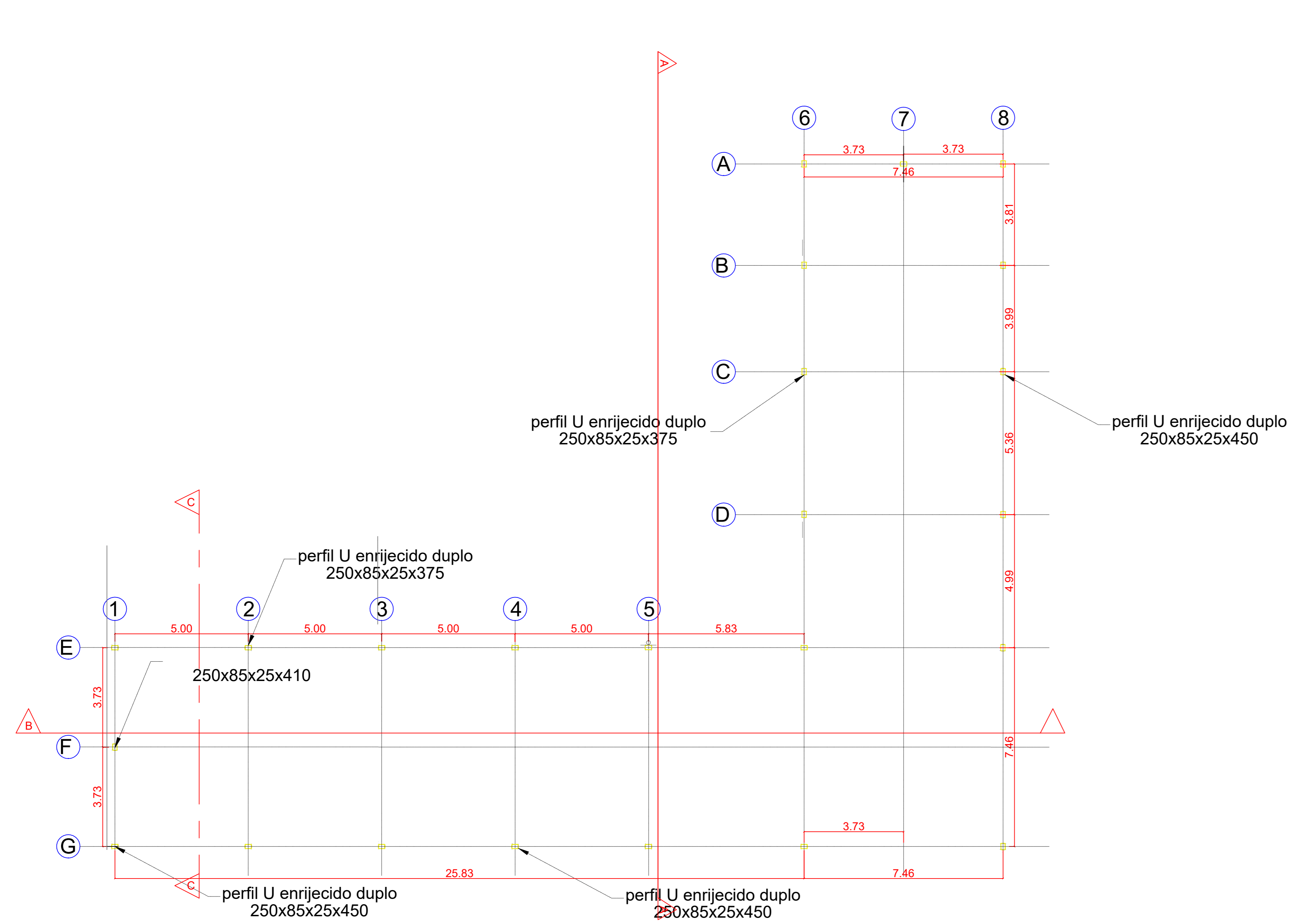
1 LOCAÇÃO DE PILARES ESCALA -1 : 100
